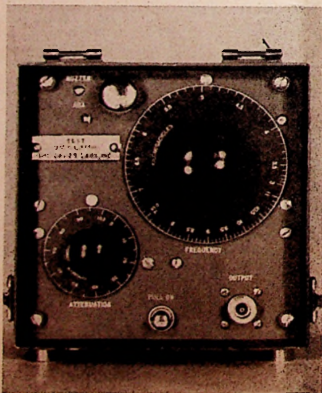
Fig. 3 De zoemergolfmeter voor golflengten tot 1 cm. De straal is geijkt in frequenties in kilomegahertz.
