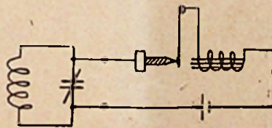
Fig. 1 Zoemergolffmeter met L C-kring
